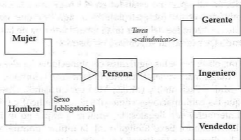
Figura 5-2: Clasificación dinámica
