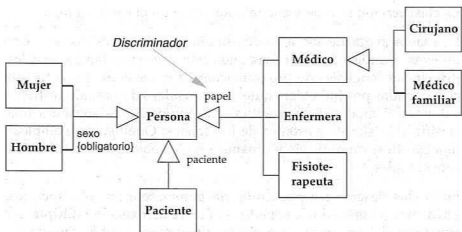
Figura 5-1: Clasificación múltiple
